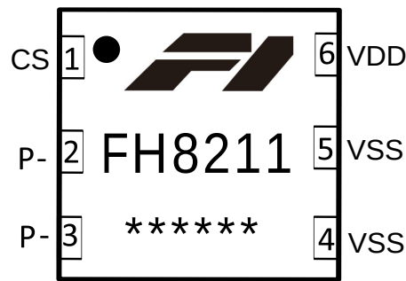
图 1 FH8211 管脚排列图（顶部视图，不成比例）
