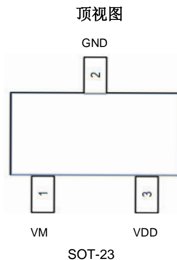
图 1. 引脚定义图
